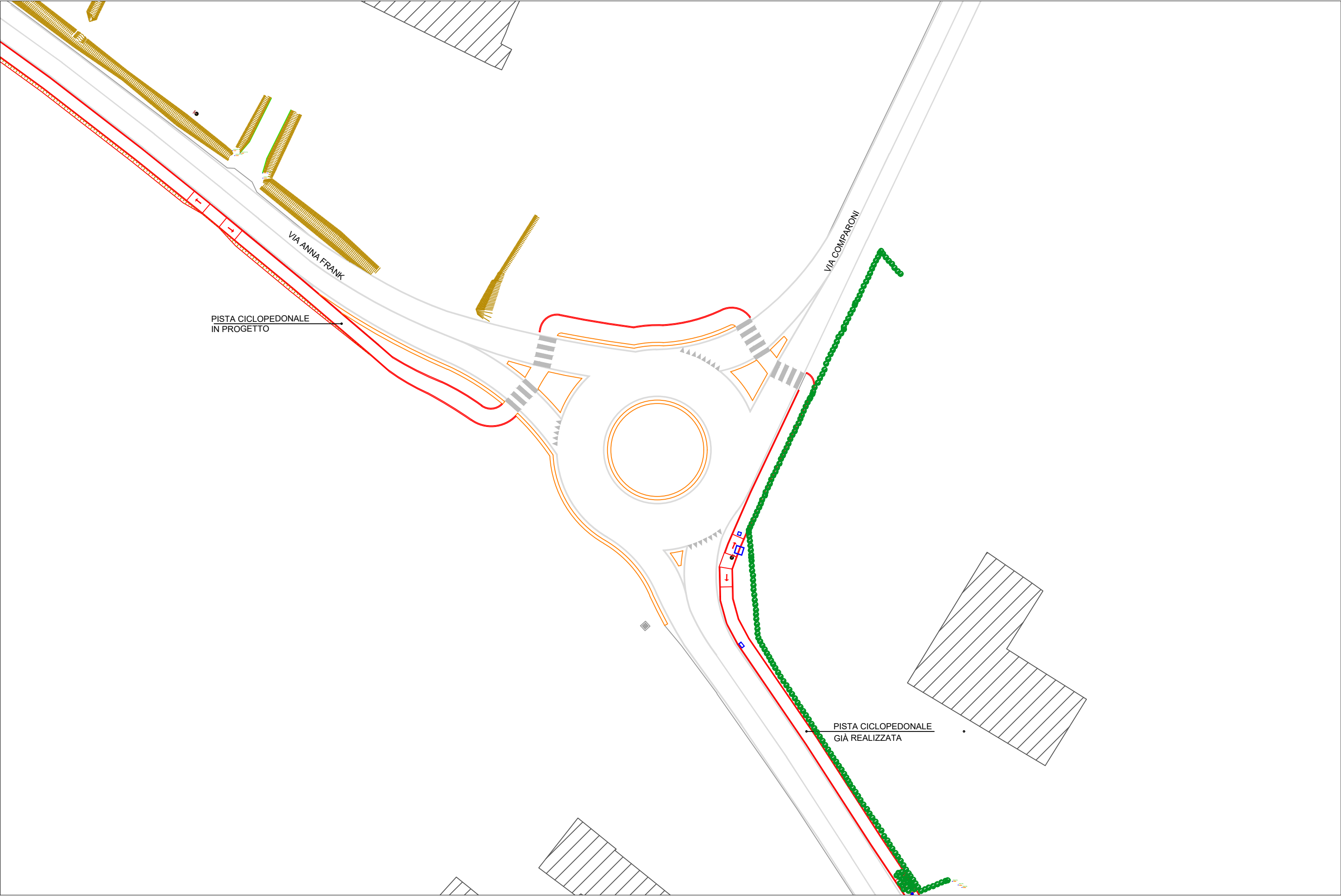
Allegato A - Schema rotatoria
