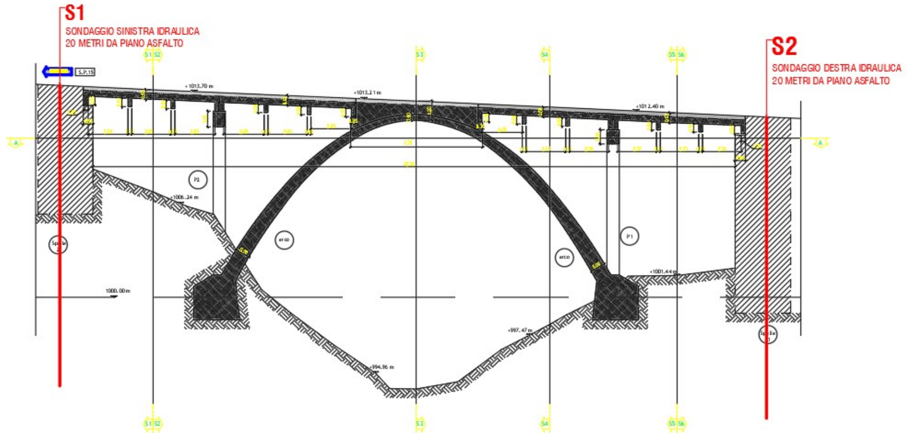
Fig.1 – Sezione schematica relativa al posizionamento delle verticali di sondaggio S1 e S2
