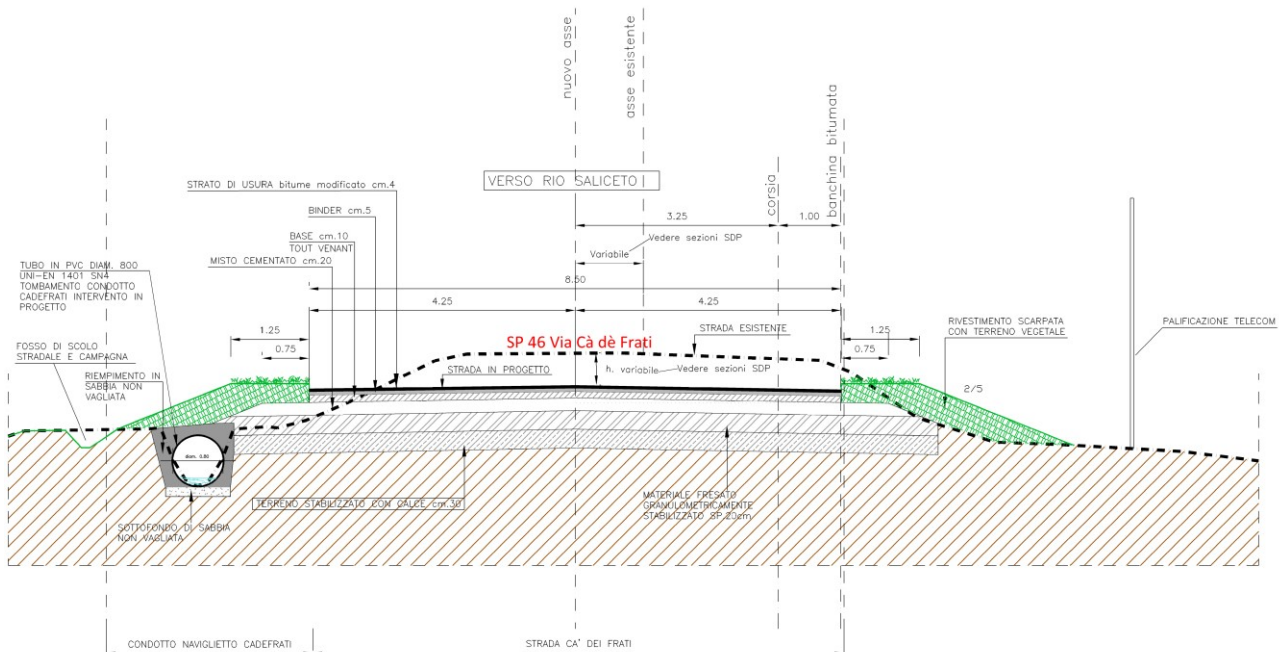
Figura 1 – Sezione tipologica di progetto (lato Rolo)
