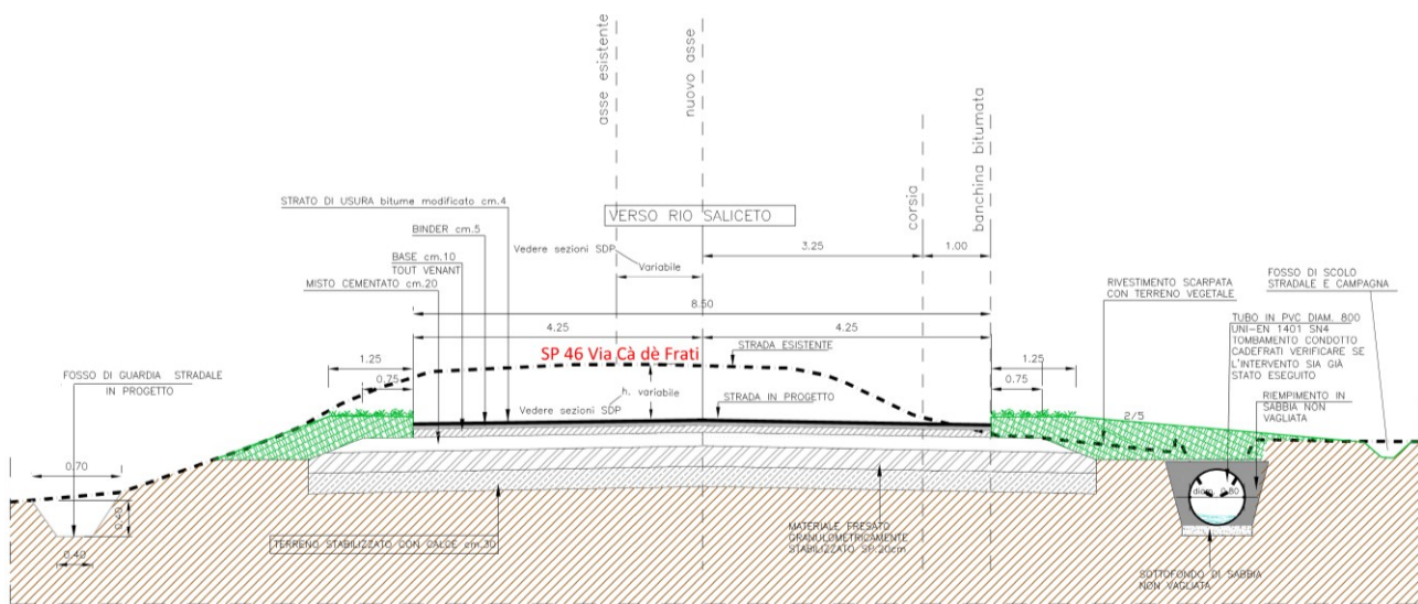
Figura 2 – Sezione tipologica di progetto (lato Rio Saliceto)
