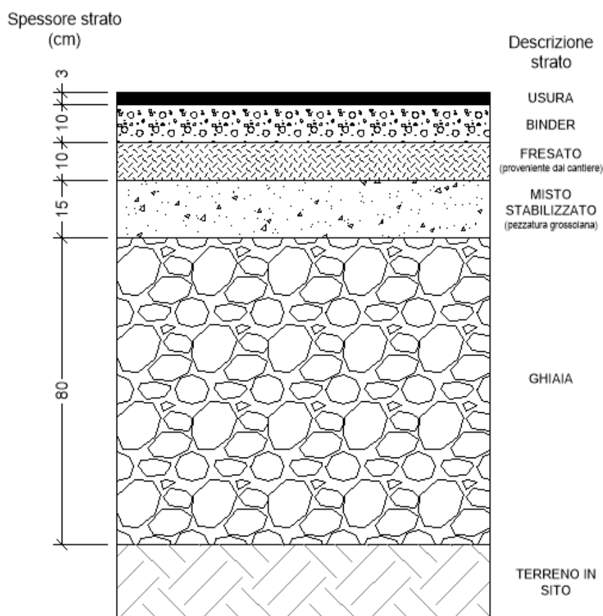
Fig. 3 – Sezione tipo 2 di risanamento del corpo stradale nel caso della carenza di capacità portante del sottofondo.
