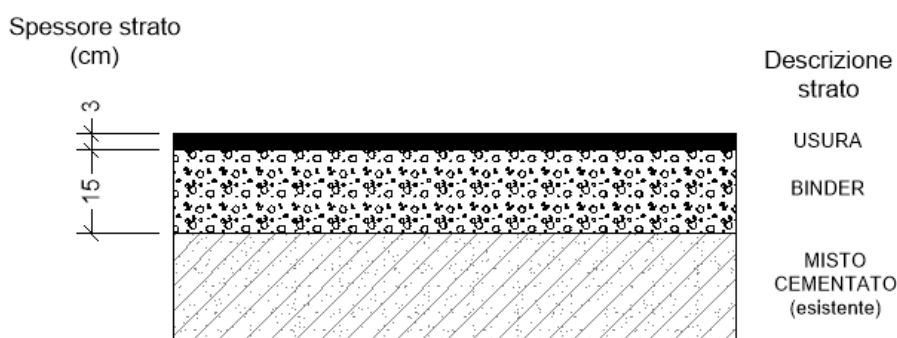
Fig. 4 - Sezioni tipo 3 di risanamento del corpo stradale nel caso in cui sia necessario il rifacimento del solo pacchetto dei conglomerati bituminosi.
