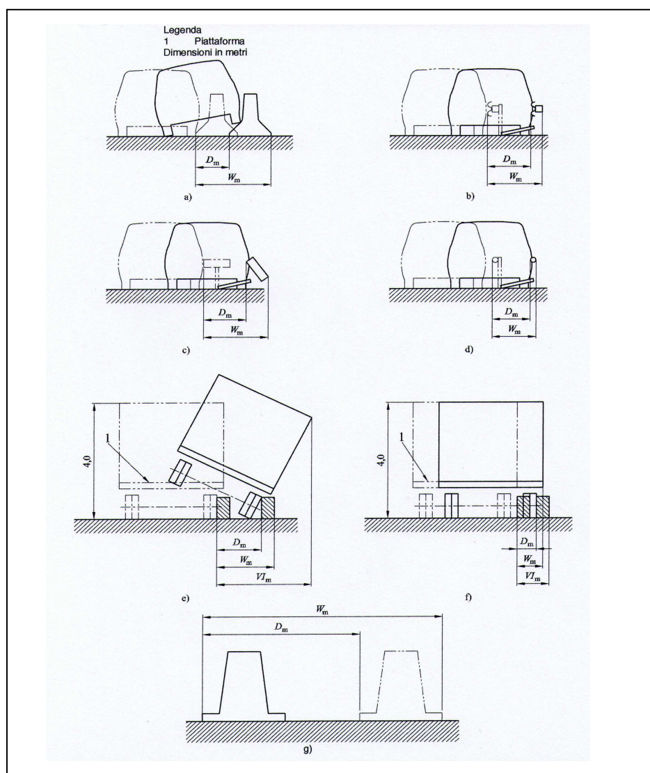
Fig. 3.9: Deflessione Dinamica D_m , Larghezza Operativa W_m e Intrusione del veicolo VIm .
